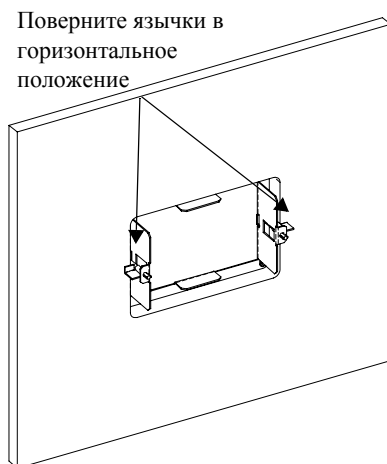
Рис. 2-5 Крепление монтажной пластины
