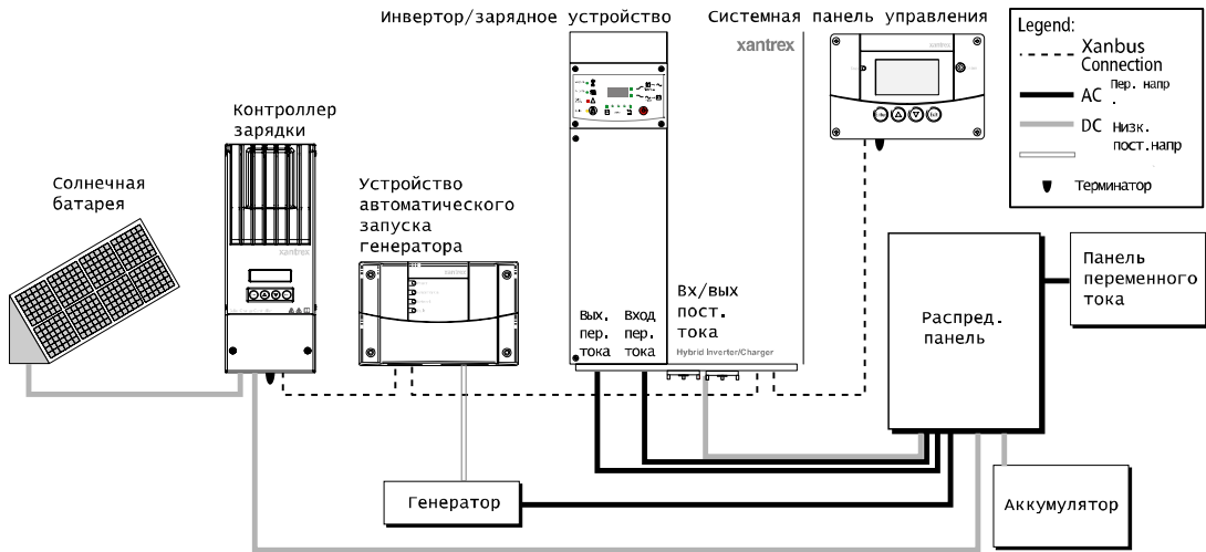
Рис. 1-3 Схема сети Xanbus
